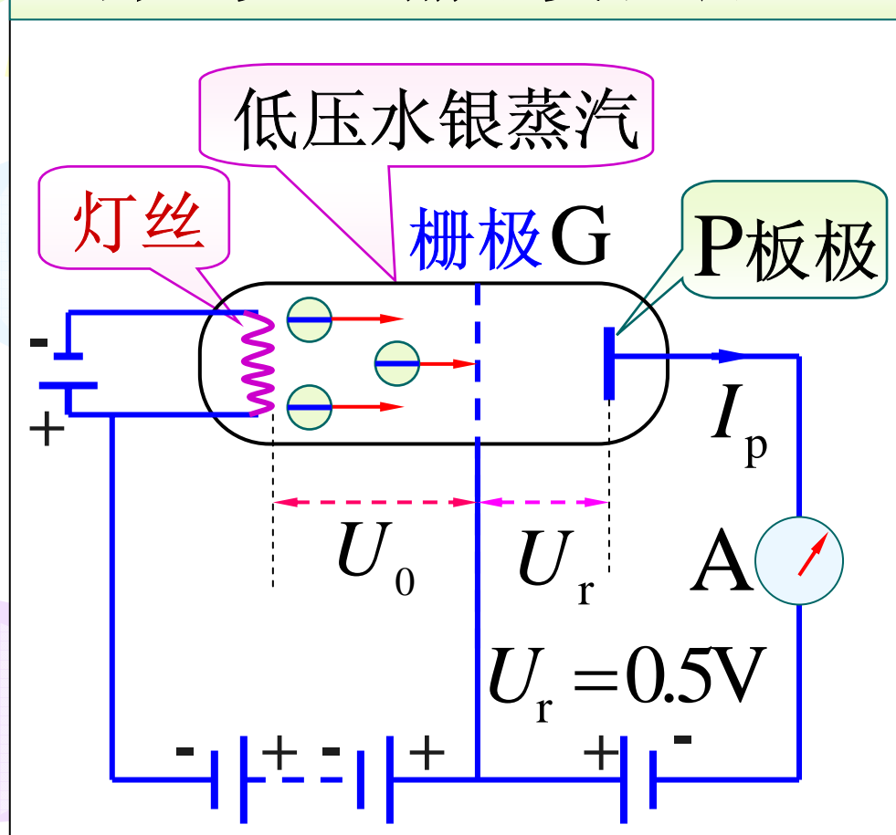
弗兰克 — 赫兹实验装置
