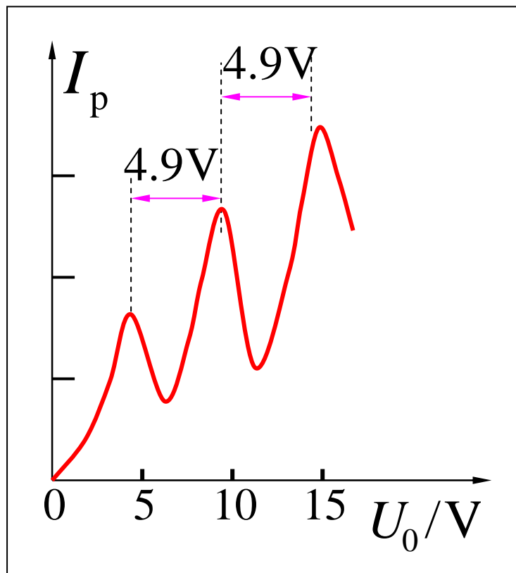
板极电流和加速电压之间的关系
